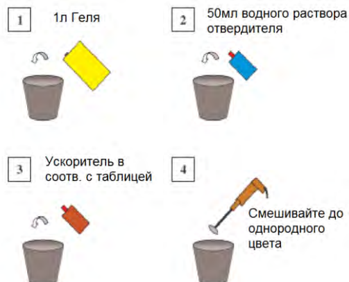
Рис. 1 - Смешивание компонентов состава.
